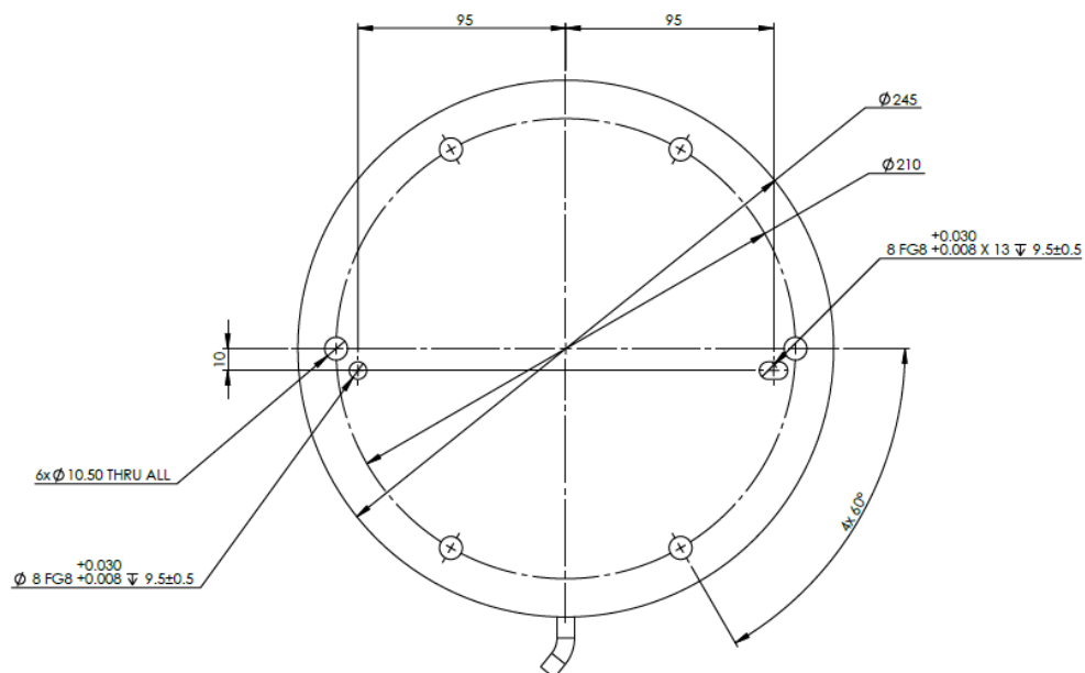
1.1: Vista inferior de la base del robot
